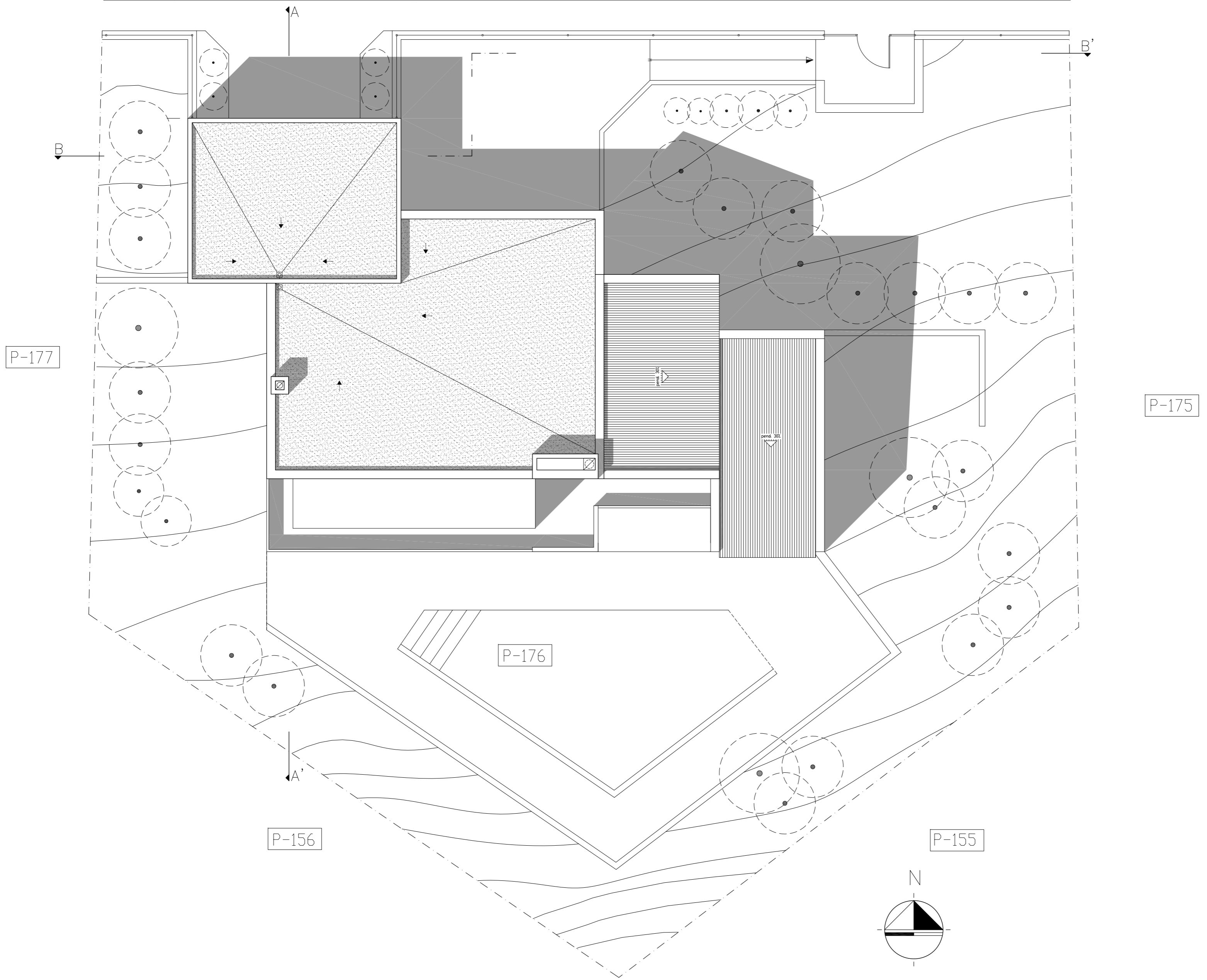
PLANO EMPLAZAMIENTO Y CUBIERTA
