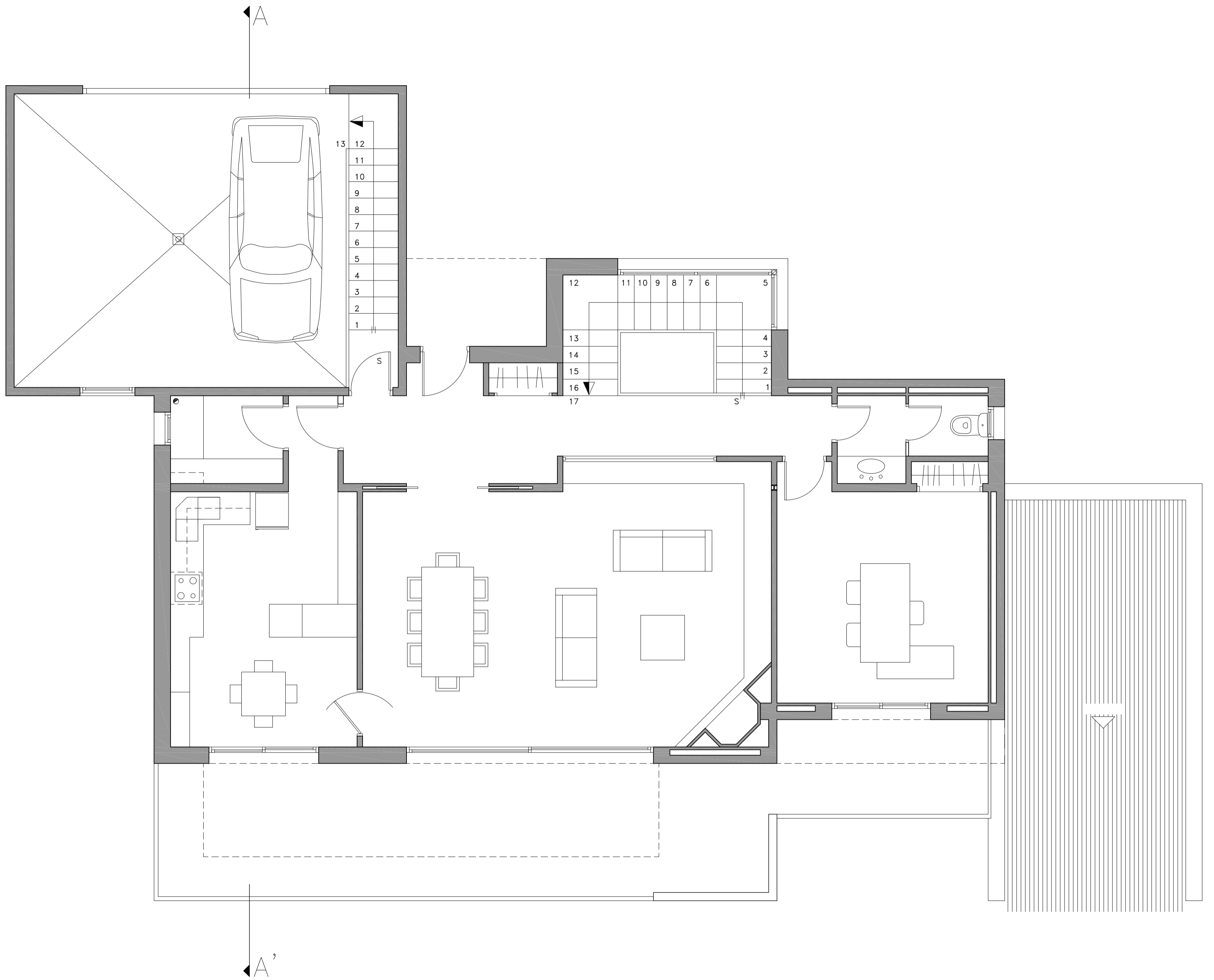
PLANTA PISO
