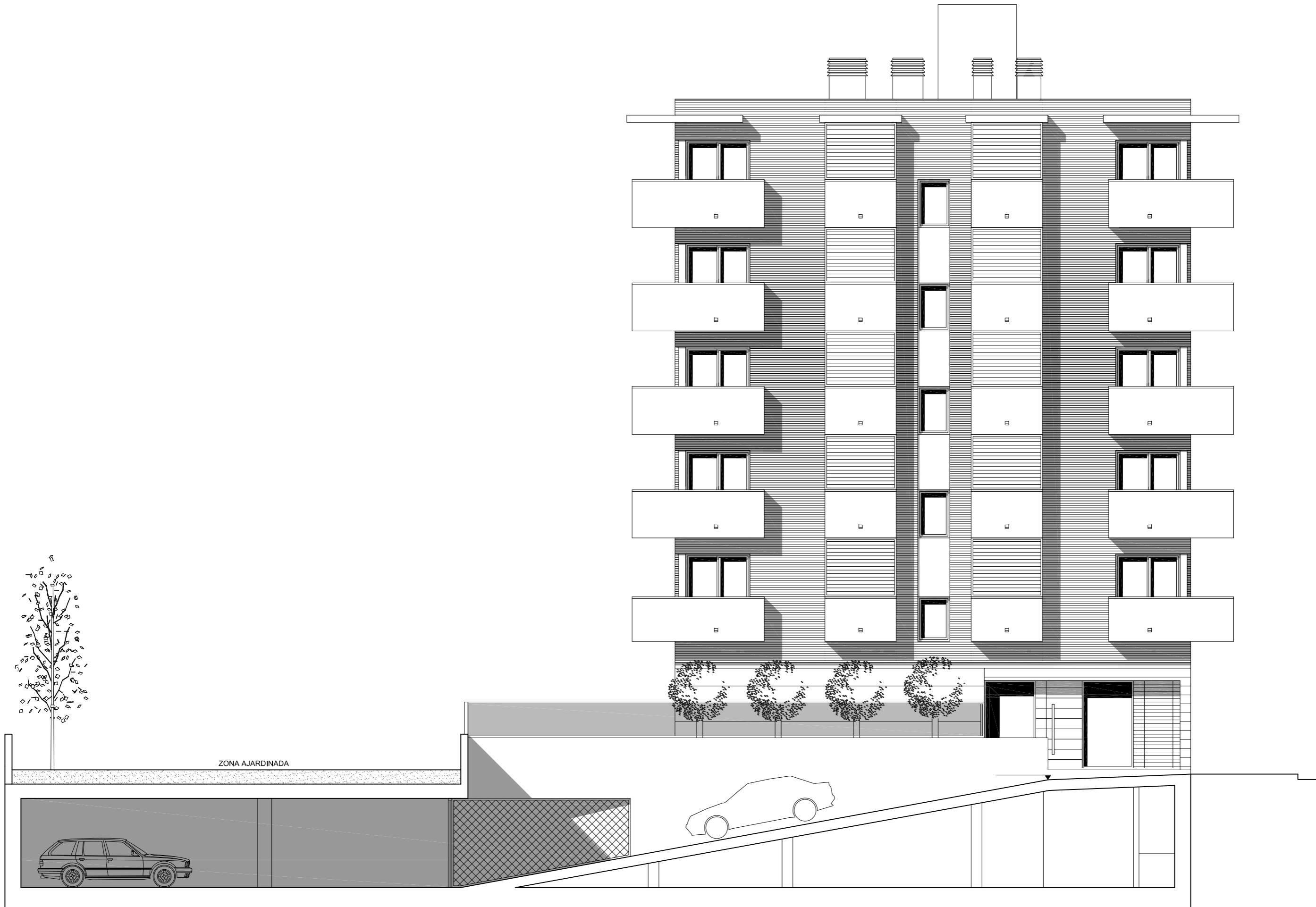
FACHADA NORTE
