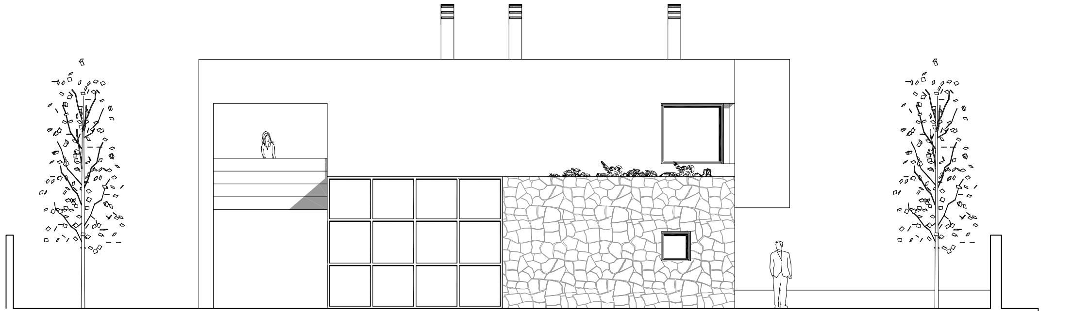
FACHADA NORTE
